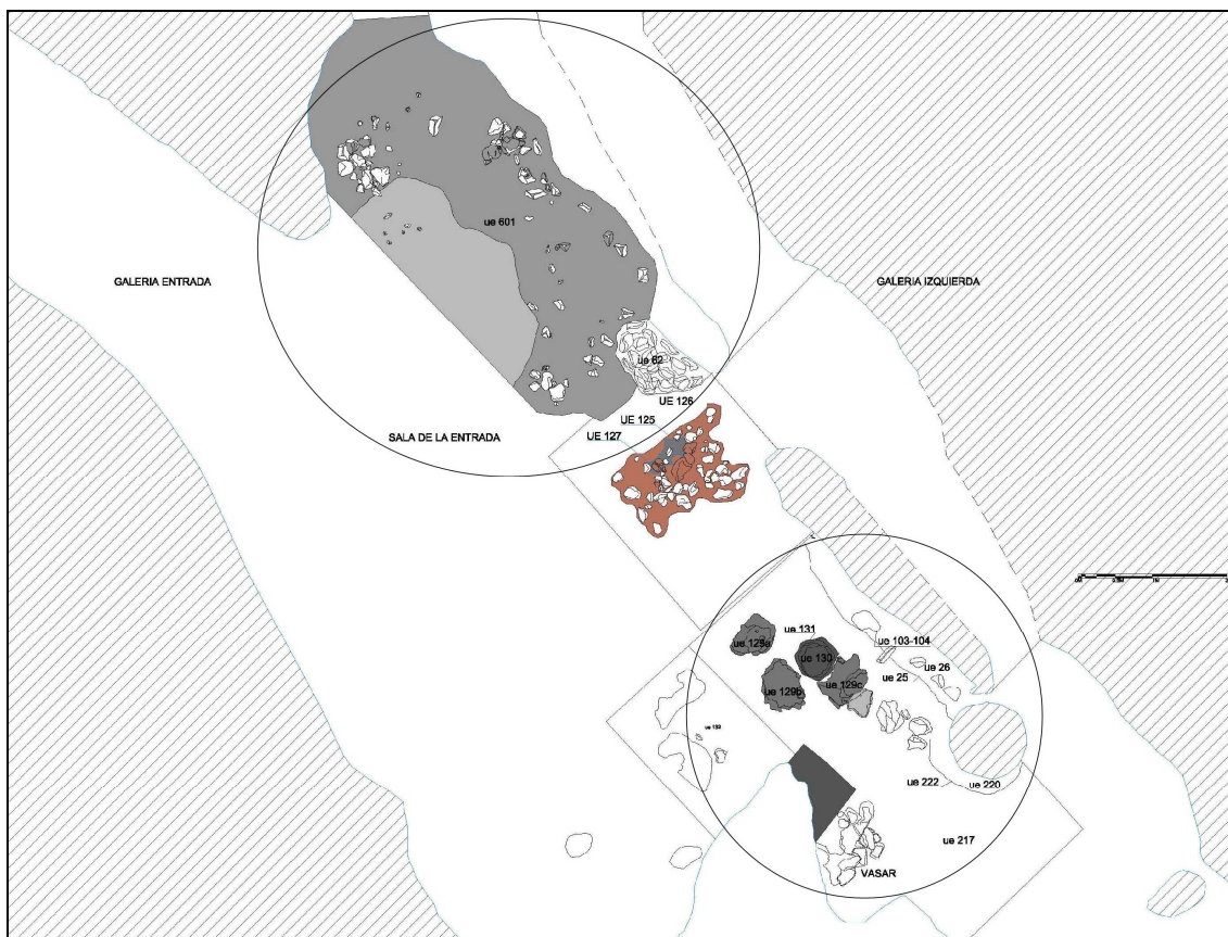
Plano de planta de la Cova del Randero.
