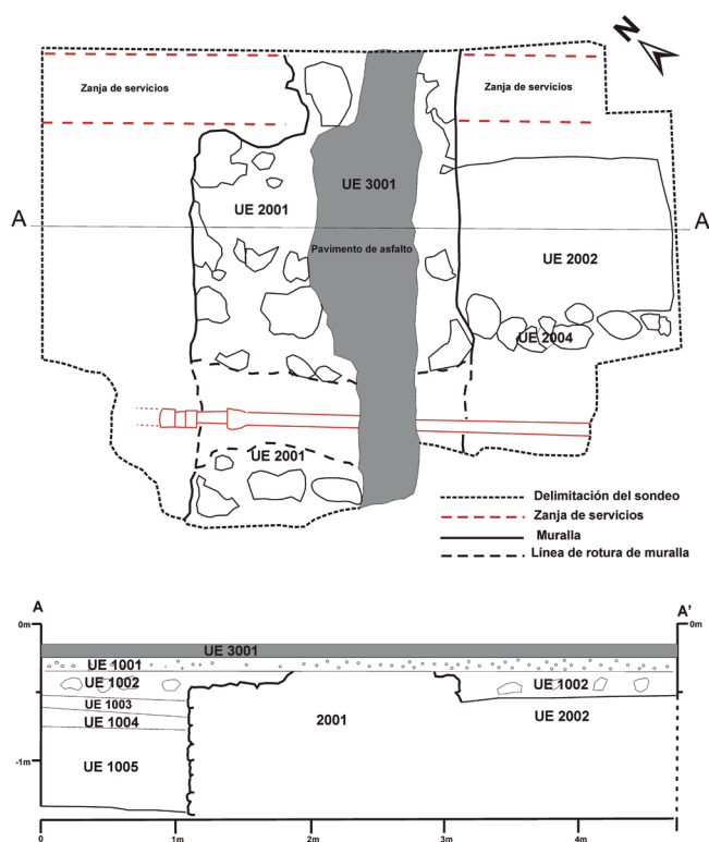
Figura 4. Planta y sección del sondeo donde aparecieron los restos de la muralla.
