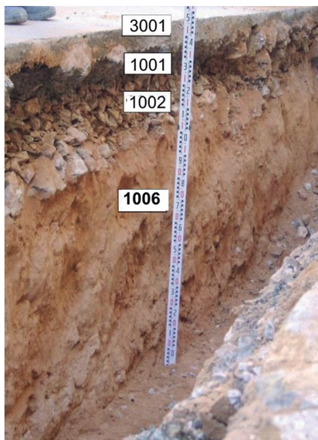
Figura 2. Estratigrafía de la zanja longitudinal abierta en la calle Ramón y Cajal.
